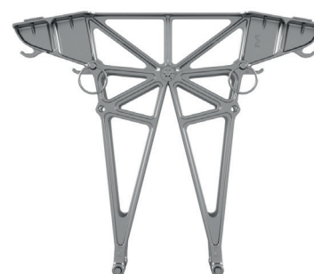
Středová vzpěra 10-15° pro jižní orientaci
