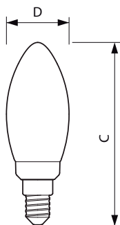
Candle B35 EU 3.5-40W 475lm WG E14 CL
