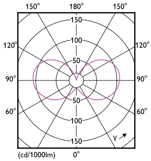
LEDbulb SSW B35 5W E14 827 CL-LDD
