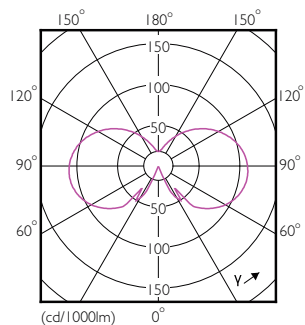
LEDbulb 40W E14 827 FR B35
