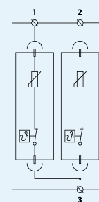
Schéma zapojení
