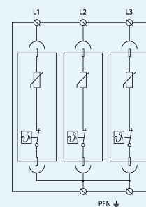
Schéma zapojení
