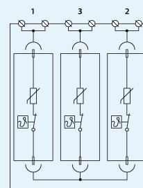
Schéma zapojení
