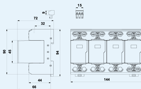
Rozměry produktu
