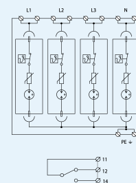
Schéma zapojení
