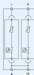
Schéma zapojení
