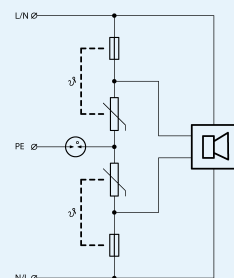
Schéma zapojení
