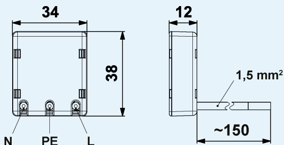
Rozměry produktu
