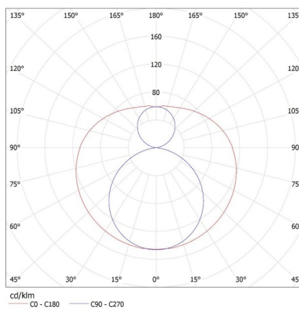
MILED0 (kat 31191) T8 N LED 18W-NW / LDC (Polar)
