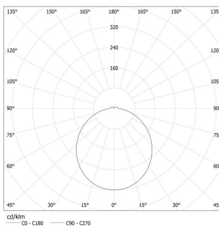
KANLUX S.A. (kat 26446) VARSO LED 24W-WW-L / Krzywa rozsyłu światła (biegunowo)
